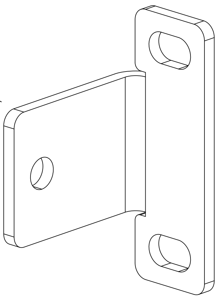
Kovový držák pro montáž výplně brány a branky
