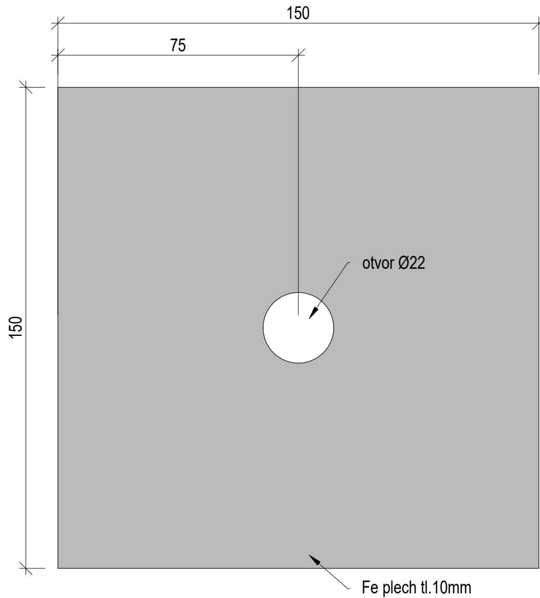
Ocelová plotna 150x150x10mm
