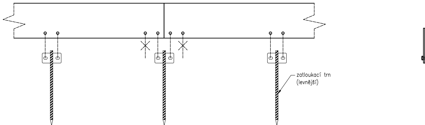
Obrubník s montážními otvory
