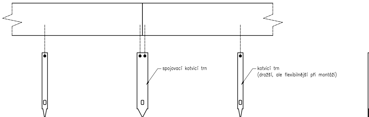
Obrubník bez montážních otvorů
