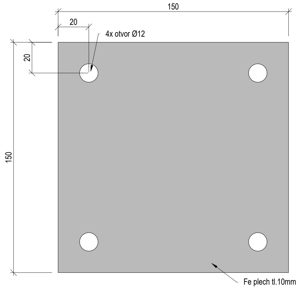
Ocelová plotna 150x150x10mm
