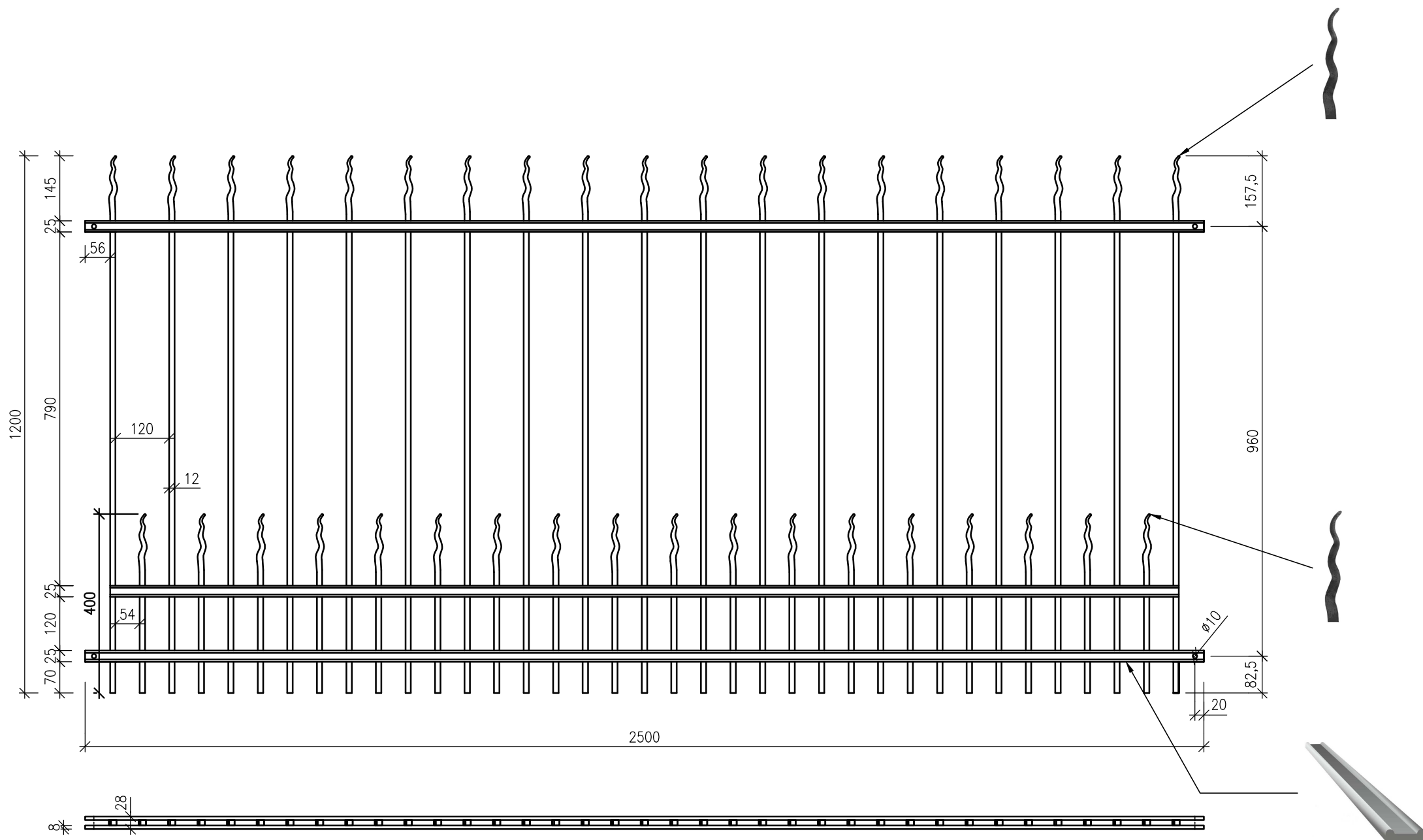
Kovové plotové pole PLP20 - š. 2500 x v. 1200 mm
