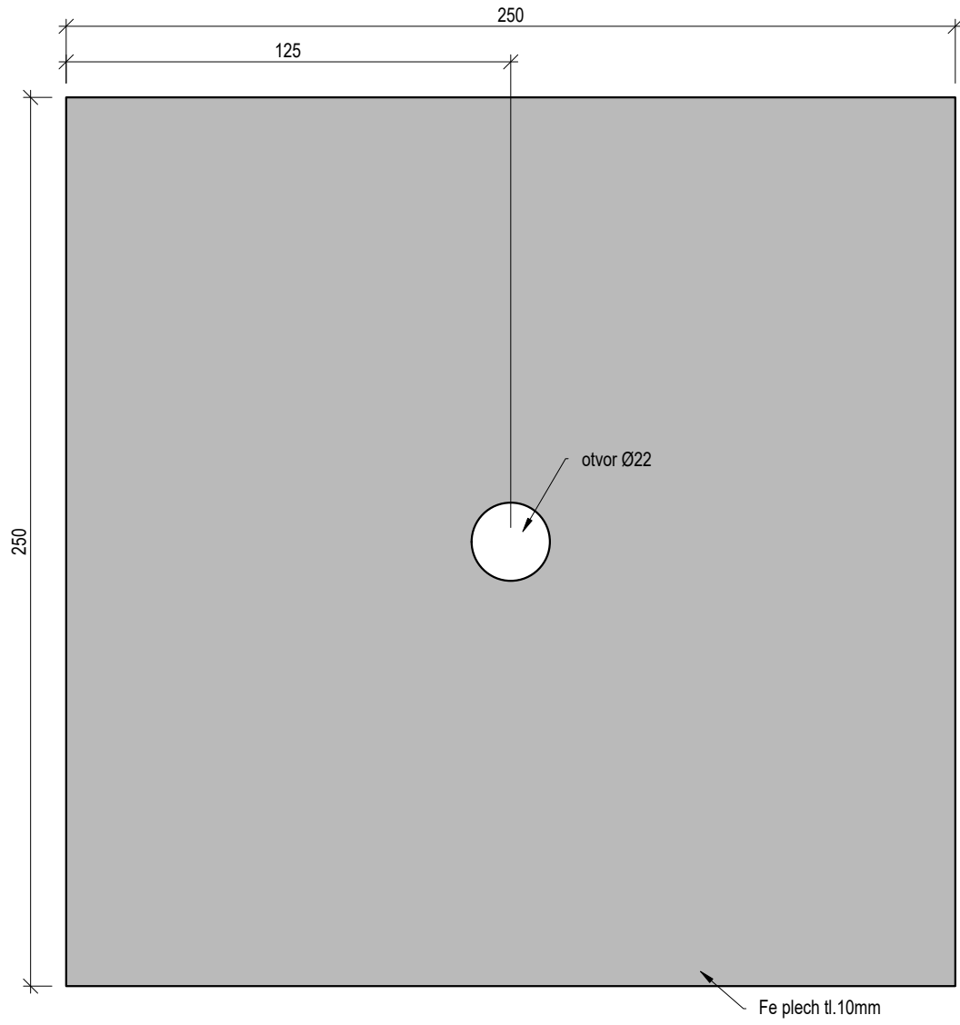
Ocelová plotna 250x250x10mm
