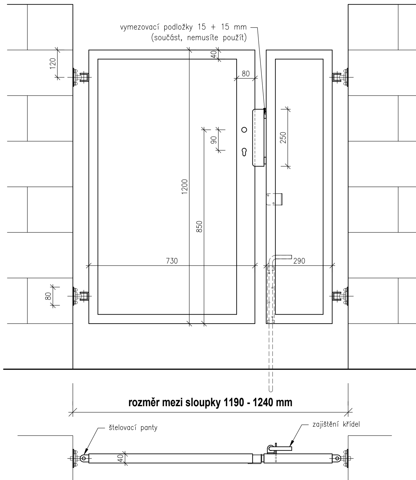
Vstupní dvoukřídlá branka š. 120 x v. 120 cm
