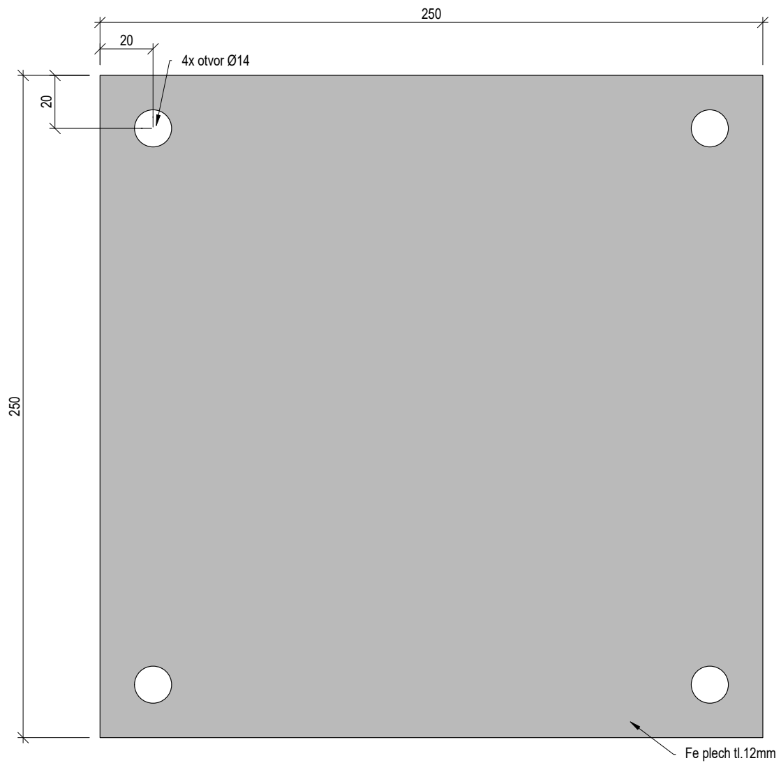
Ocelová plotna 250x250x12mm
