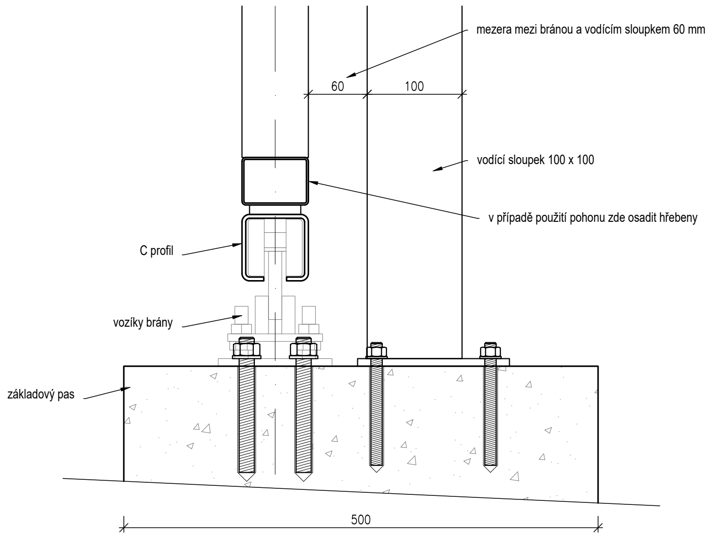
DETAIL 2 - ODSAZENÍ VODÍČÍHO SLOUPKU OD BRÁNY
