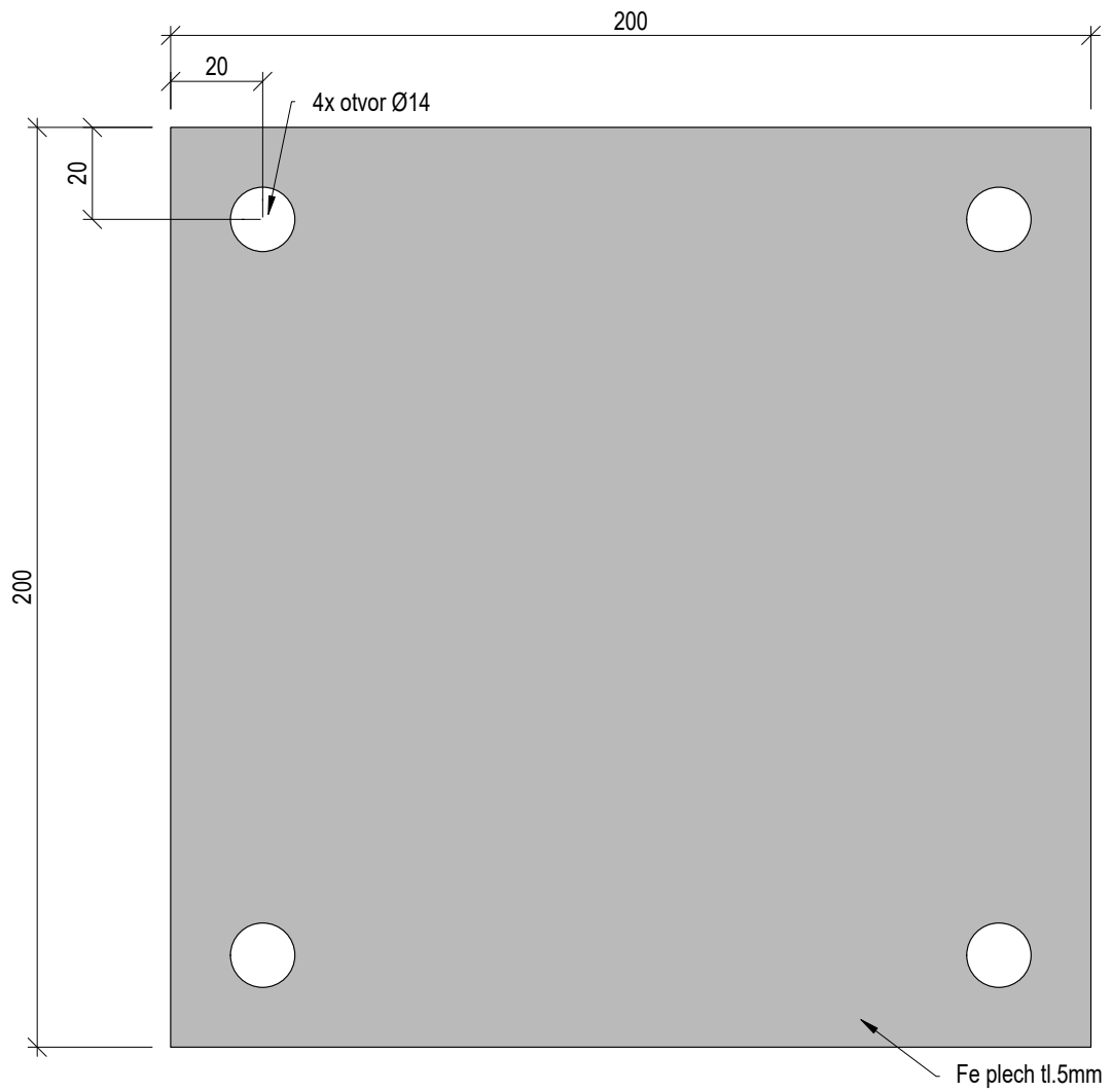
Ocelová plotna 200x200x5mm
