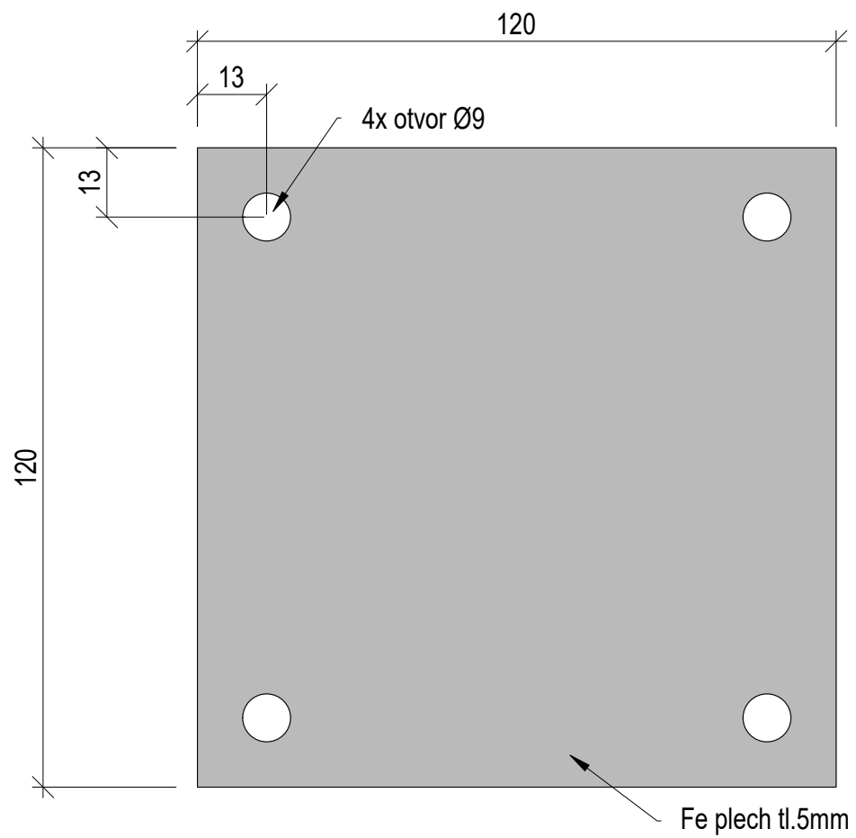
Ocelová plotna 120x120x5mm
