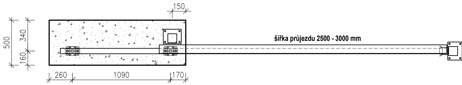
Základ samonosné posuvné brány š. 250 - 300 cm x v. 170 cm
