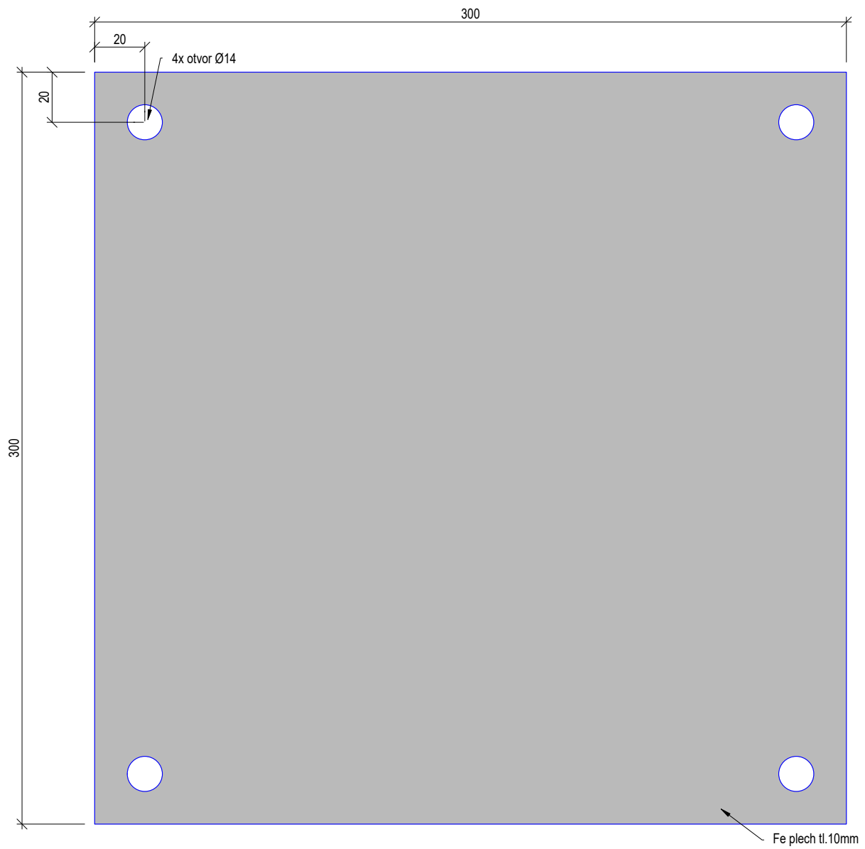
Ocelová plotna 300x300x10mm
